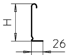
Размеры
