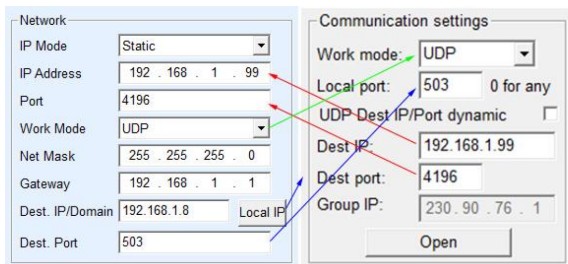
Chart 19 UDP mode parameter configuration
