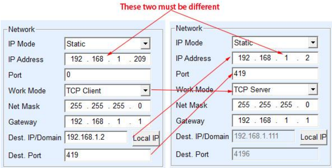
Chart 20 TCP device pairing parameter configuration
